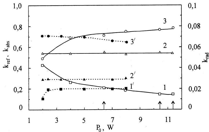
Рис. 2. Энергетические характеристики СВЧ-разрядов.
